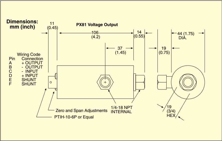
STANDARD PX81D0-100D5T, shown actual size.
