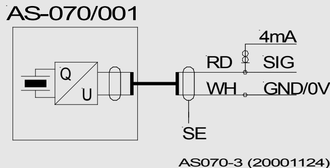
Fig. 3 Wiring diagram
