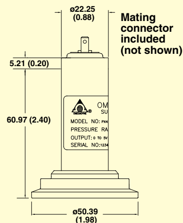
PX419S15 1½" flange
