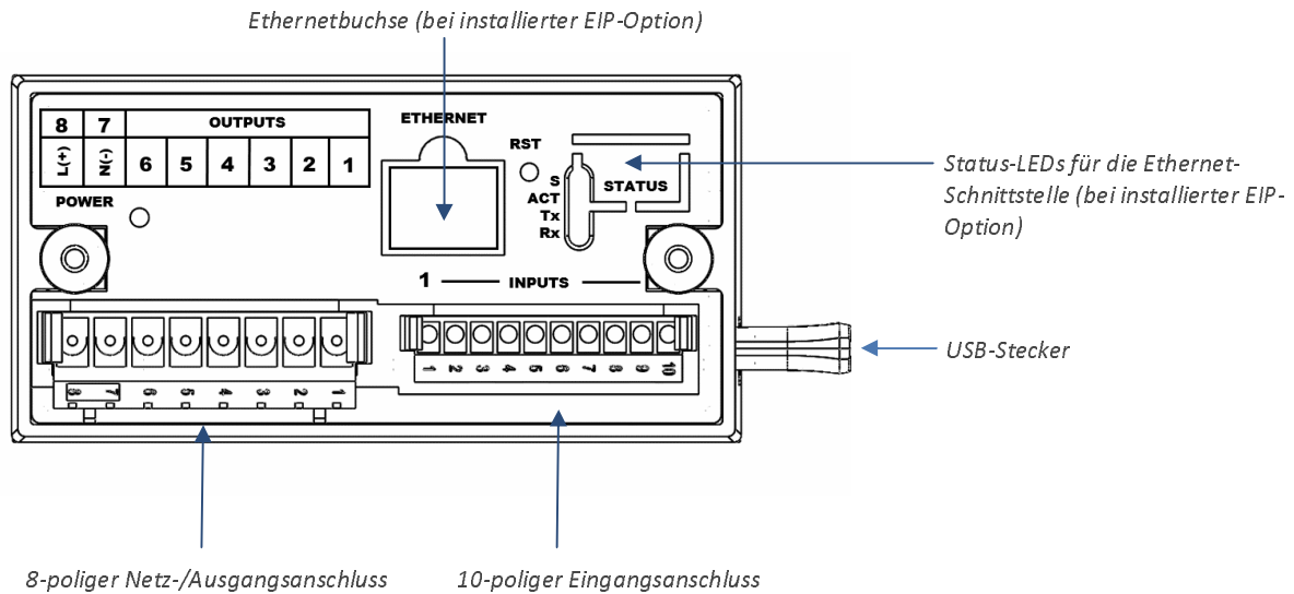
Abbildung 1 – DP8Pt-Modelle: Anschlüsse auf der Rückseite
