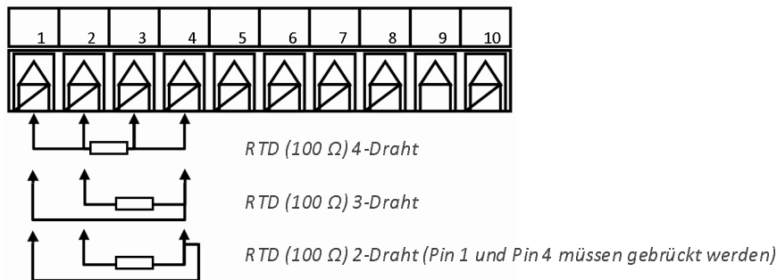
Abbildung 4 – Widerstandsfühler-Verdrahtung
