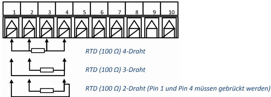
Abbildung 4 – Widerstandsfühler-Verdrahtung
