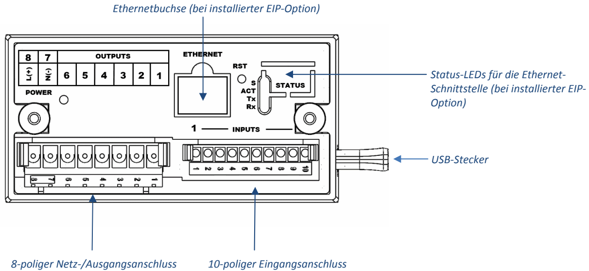
Abbildung 1 – Modelle CN8Pt: Anschlüsse auf der Rückseite
