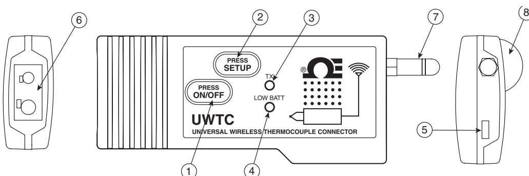
Conector de termopar (UWTC-1, UWTC-2)
