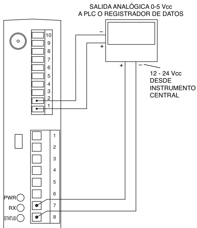
Ejemplo de salida de voltaje
