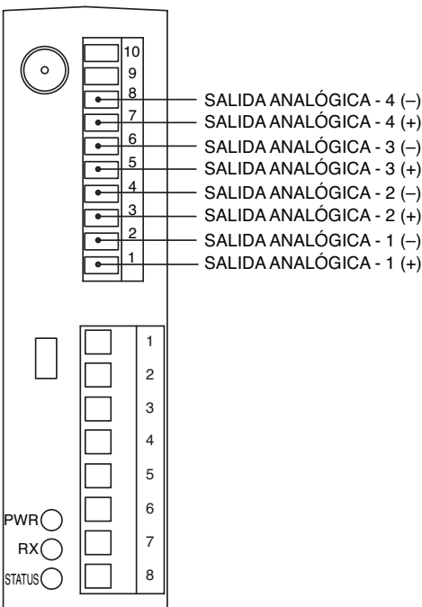
Conexiones de salida analógicas
