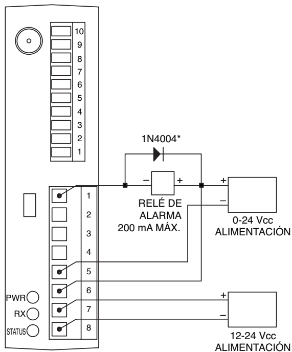
Ejemplo de alarma; alimentación externa
