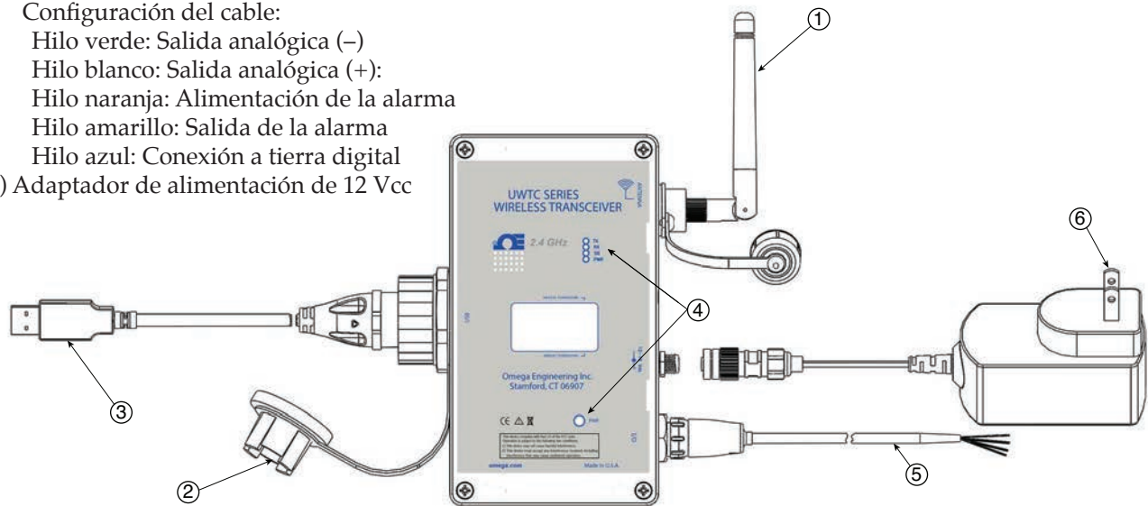
Funcionamiento del receptor. Modelo UWTC-REC2-D-*-NEMA
