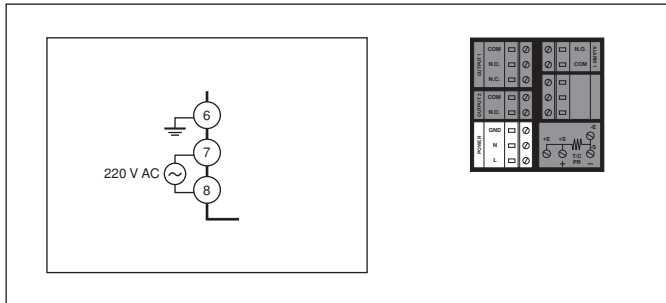
Abbildung 1-6. Spannungsversorgung
