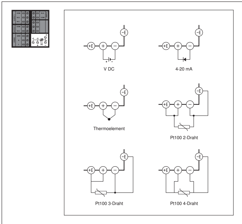
Abbildung 1-7. Verdrahtung der Eingangsklemmen
